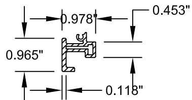
⑪ TRANSOM ALUM. REINF.-612428
